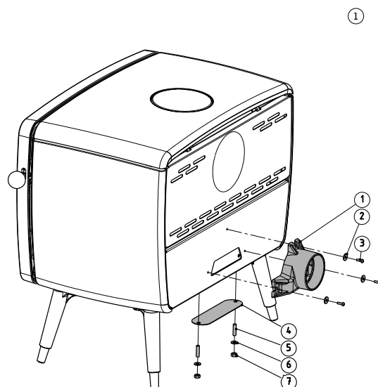
Fig. 9 Monter horisontal stuss for direkte tilførsel av forbrenningsluft som vist på skissen. Fjern mutter (7) og skive (6) og monter dekkplaten (4). Monter deretter stussen (1) med skiven (2) og skruen (3).
