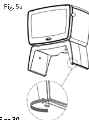
5a Justering/vatring av Tablet, Woodbox og Cradle
