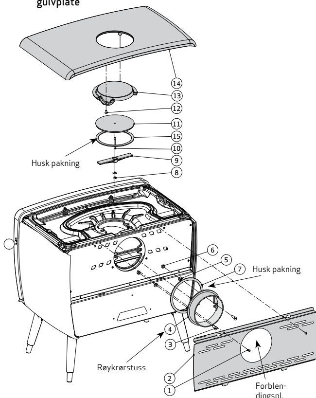
Fig. 6 Montering av røykuttak bak
